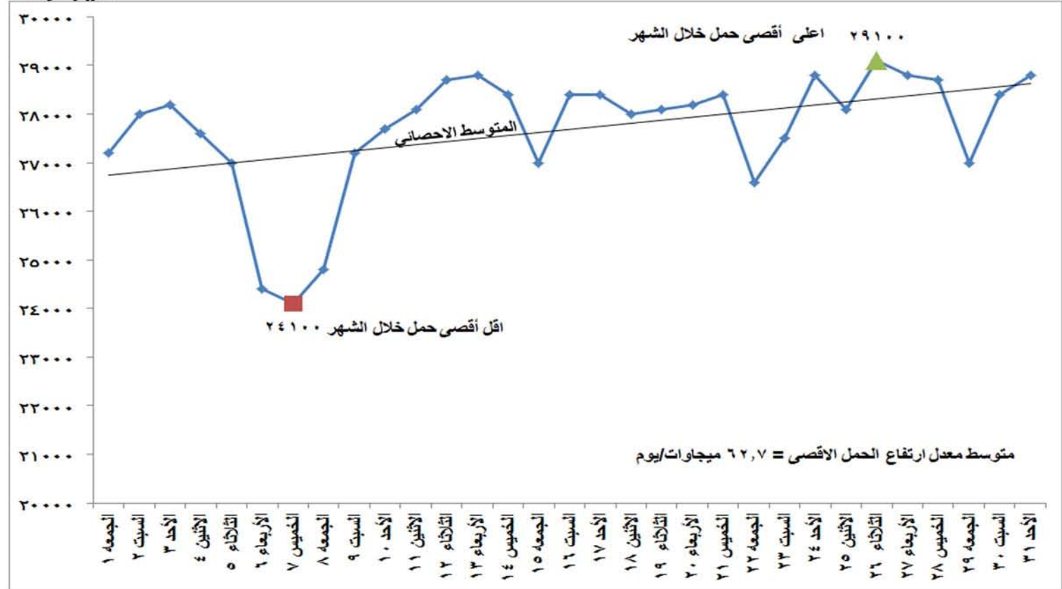
شكل (١) تطور الحمل الاقصى اليومي خلال شهر يوليو ٢٠١٦
