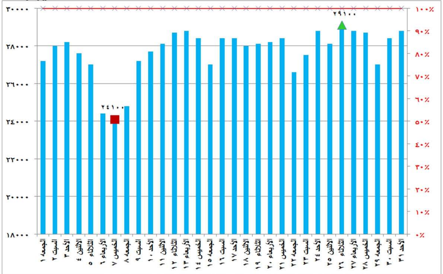
شكل (٥) قدرات الانتاج المتاحة ونسبتها للحمل الاقصى خلال شهر يوليو ٢٠١٦
