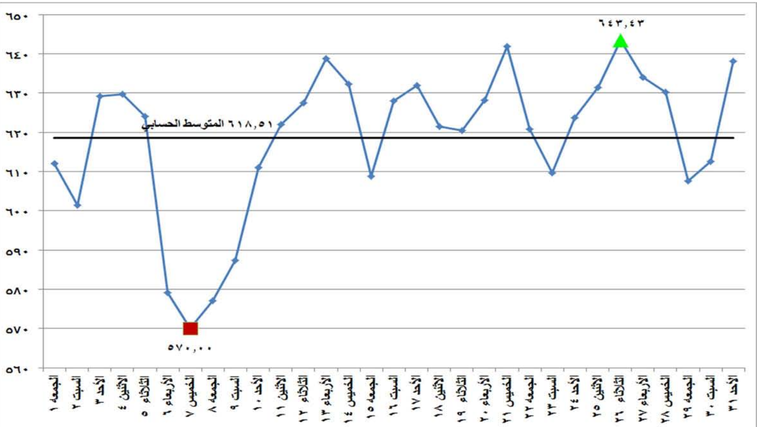
شكل (١٤) معامل انبعاثات غاز ثاني اكسيد الكربون المكافئ على مدى شهر يوليو ٢٠١٦
