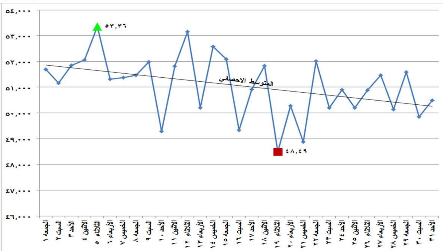
شكل (٢٣) الطاقة الكهربائية المنتجة من المصادر المائية خلال شهر يوليو ٢٠١٦
