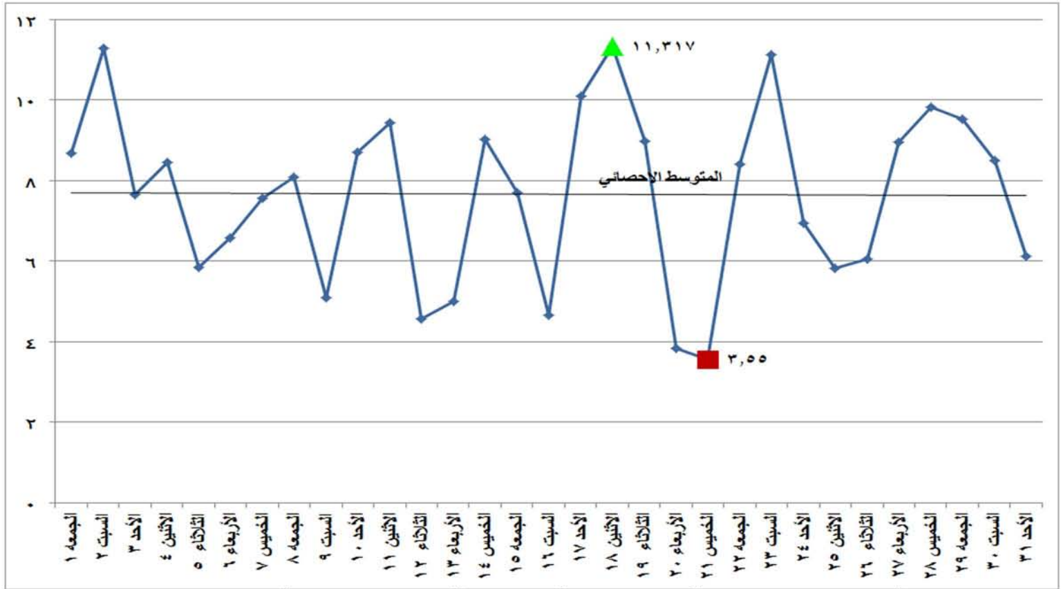
شكل (٢٥) الطاقة الكهربائية المنتجة من الرياح والشمس خلال شهر يوليو ٢٠١٦
