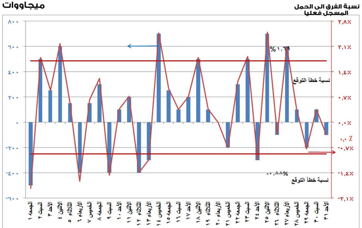
شكل (١٠) الفرق بين الحمل الأقصى المتوقع والمسجل فعلياً ونسبة الفرق إلى الحمل المسجل فعلياً خلال شهر يوليو ٢٠١٦
