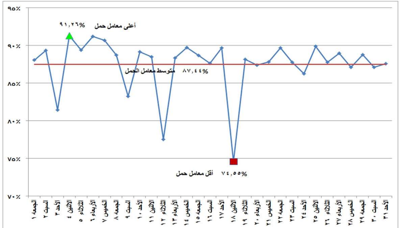
شكل (١٢) إجمالي معامل الحمل لوحدات الانتاج خلال شهر يوليو ٢٠١٦
