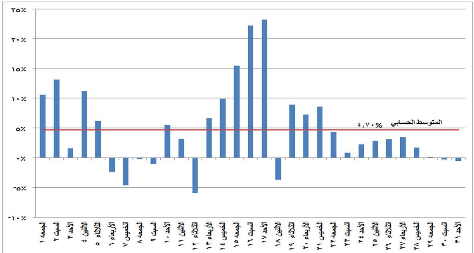
شكل (١٦) نسب التغير في الطاقة الكهربائية المنتجة خلال شهر يوليو ٢٠١٦ مقارنة بالشهر المماثل من العام السابق
