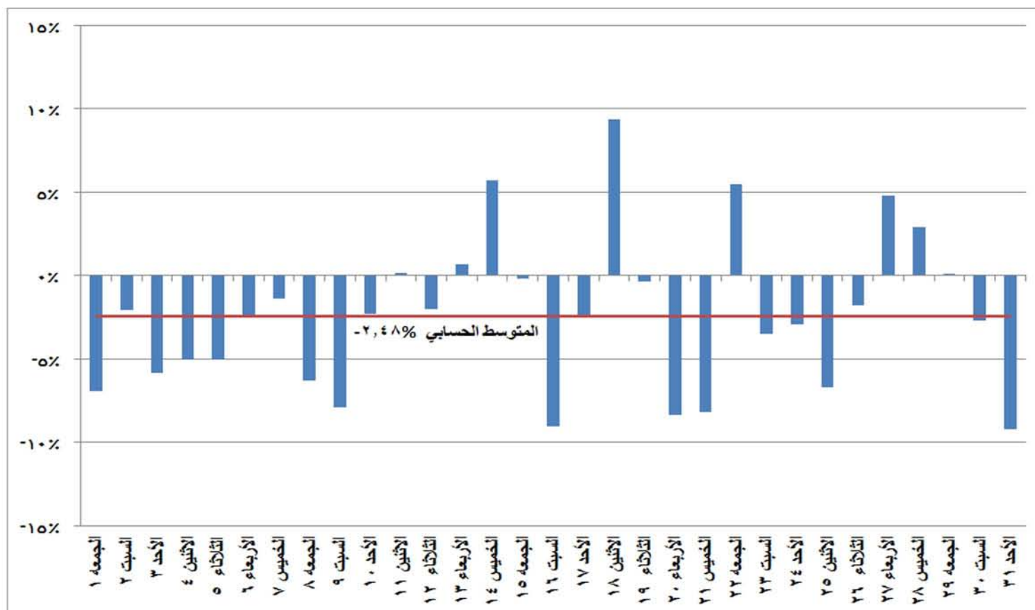
شكل (٢٢) نسب التغير في استخدام المصادر غير الحرارية في إنتاج الطاقة الكهربائية خلال شهر يوليو ٢٠١٦ مقارنة بالشهر المماثل من العام السابق
