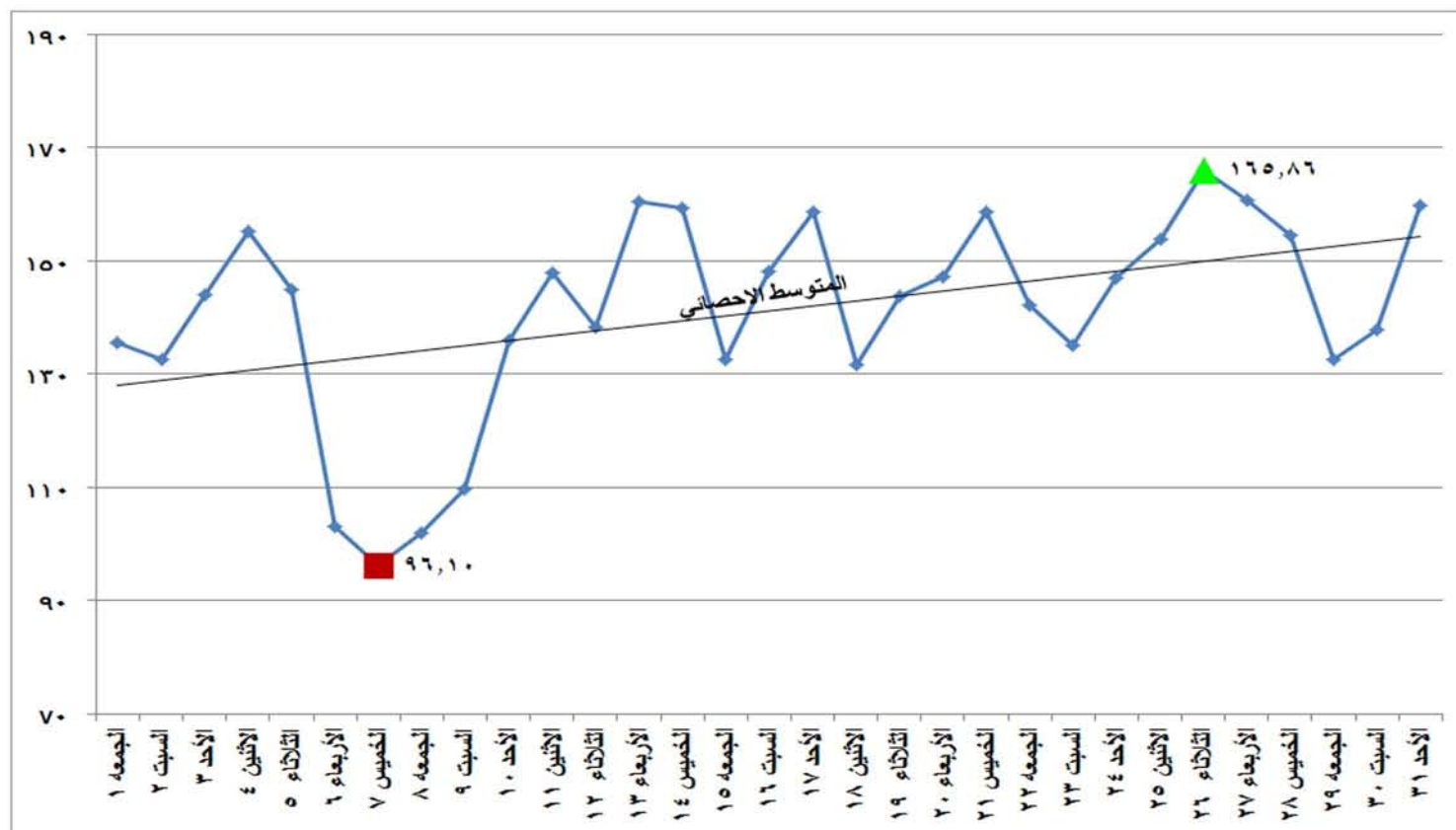
شكل (١٩) الطاقة الكهربائية المنتجة من المازوت خلال شهر يوليو ٢٠١٦
