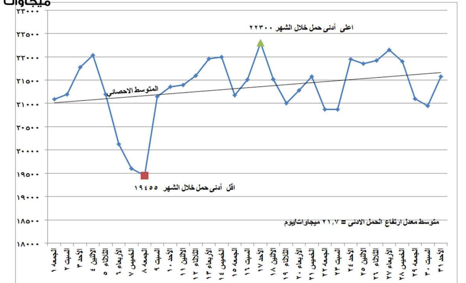
شكل (٢) تطور الحمل الأدنى اليومي خلال شهر يوليو ٢٠١٦
