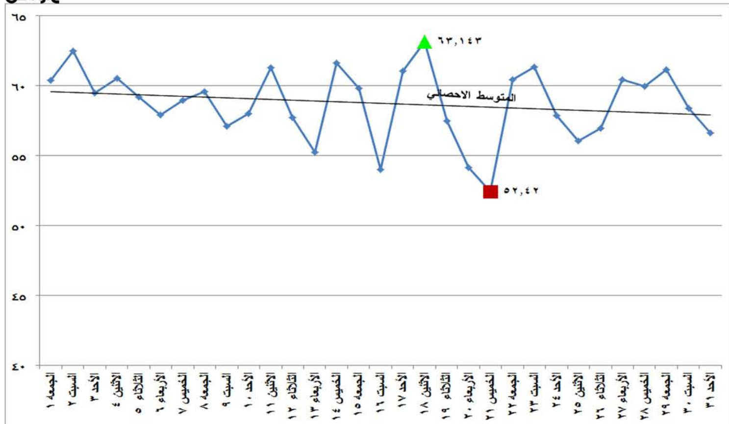
شكل (٢١) الطاقة الكهربائية المنتجة من المصادر غير الحرارية خلال شهر يوليو ٢٠١٦
