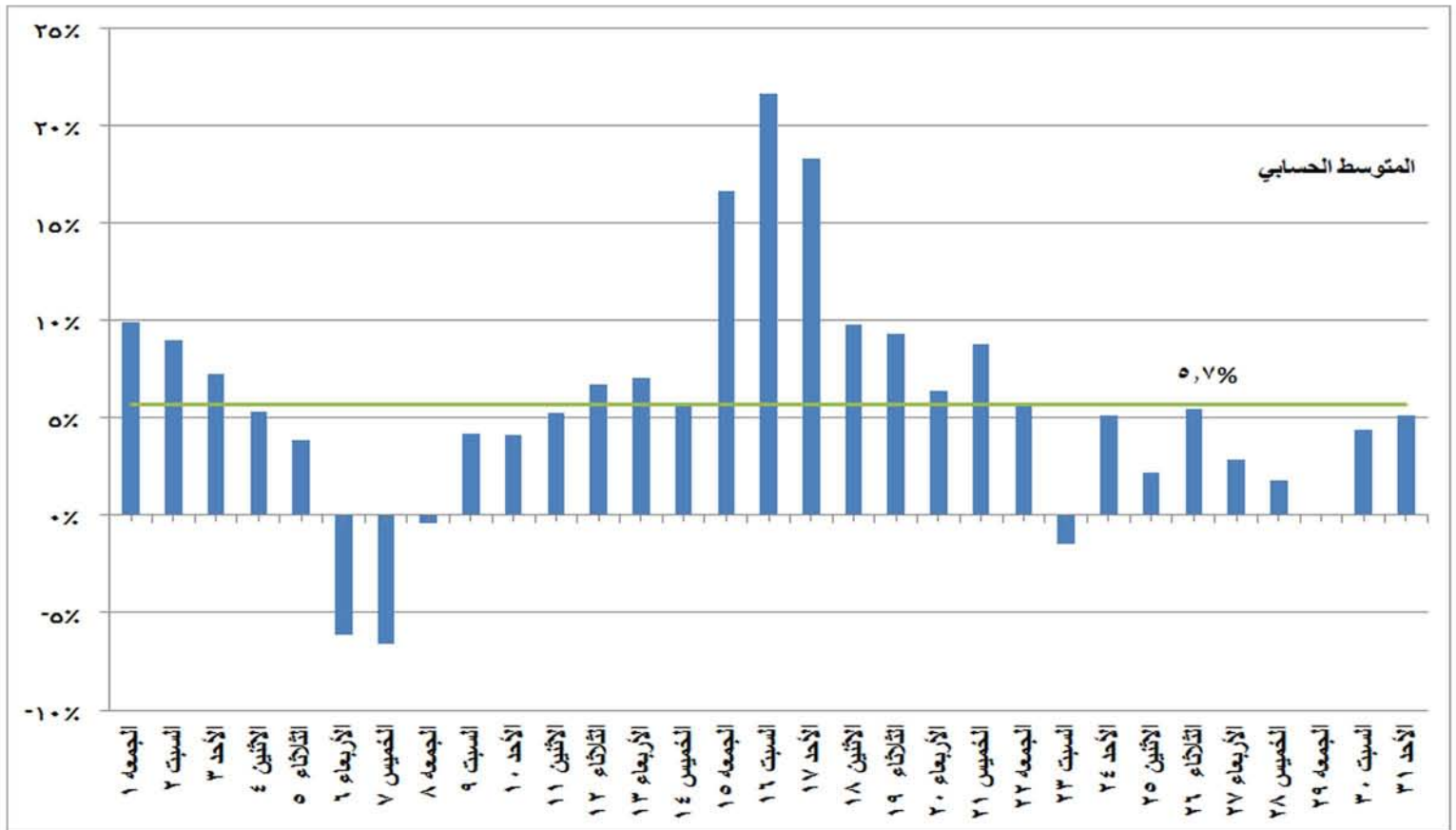
شكل (٩) النسب المئوية للتغير في الحمل الأقصى خلال شهر يوليو ٢٠١٦ مقارنة باليوم المماثل من العام الماضي
