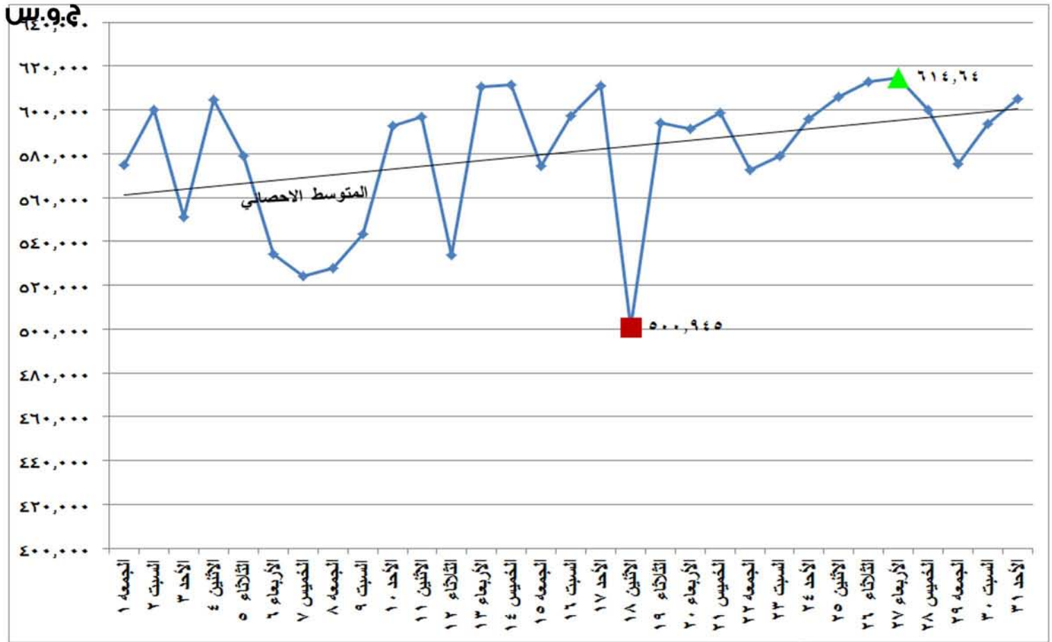
شكل (١٥) أجمالي الطاقة الكهربائية المنتجة من كل المصادر الأولية خلال شهر يوليو ٢٠١٦
