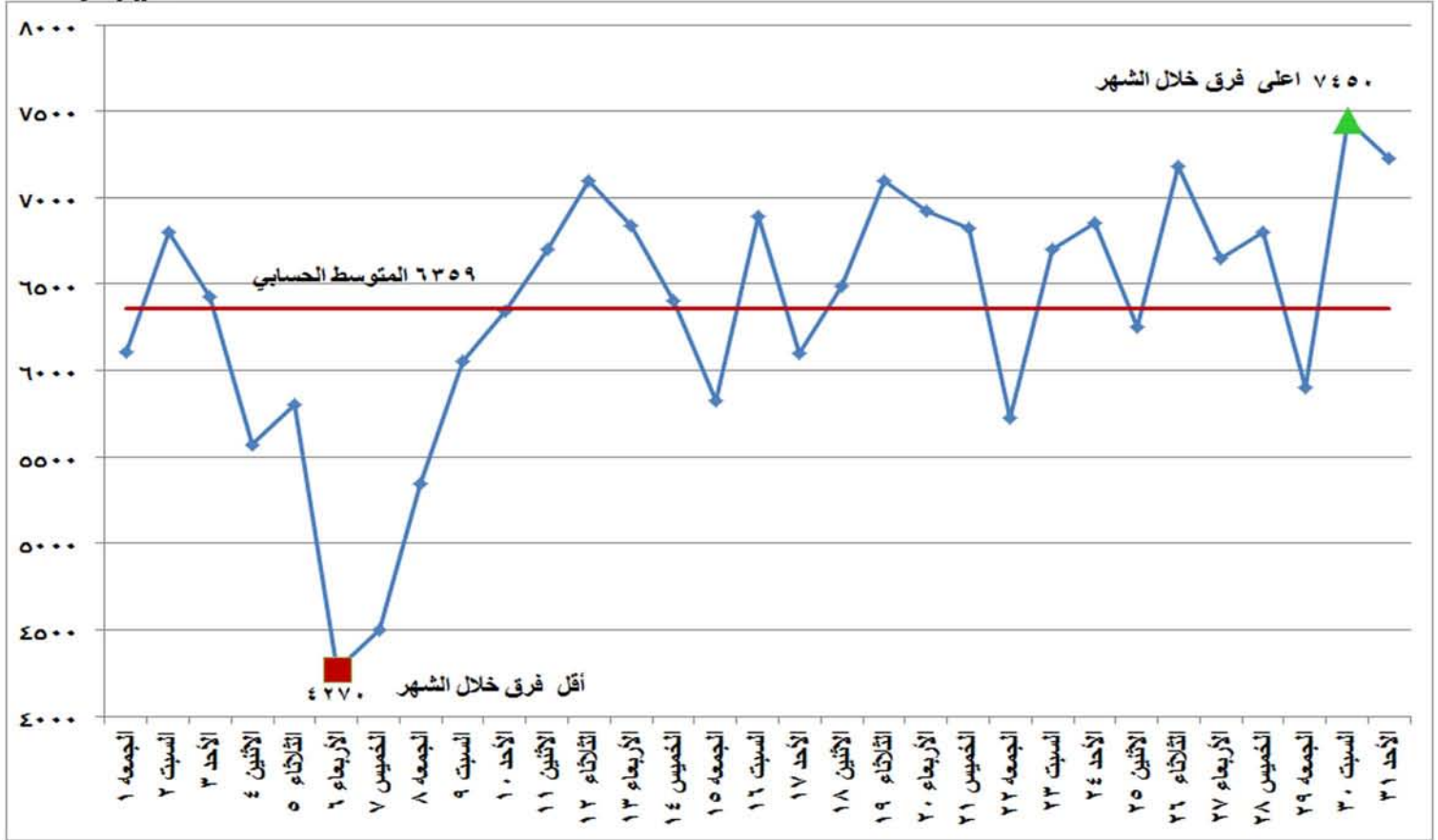
شكل (٣) الفرق بين أقصى وأدنى حمل خلال شهر يوليو ٢٠١٦
