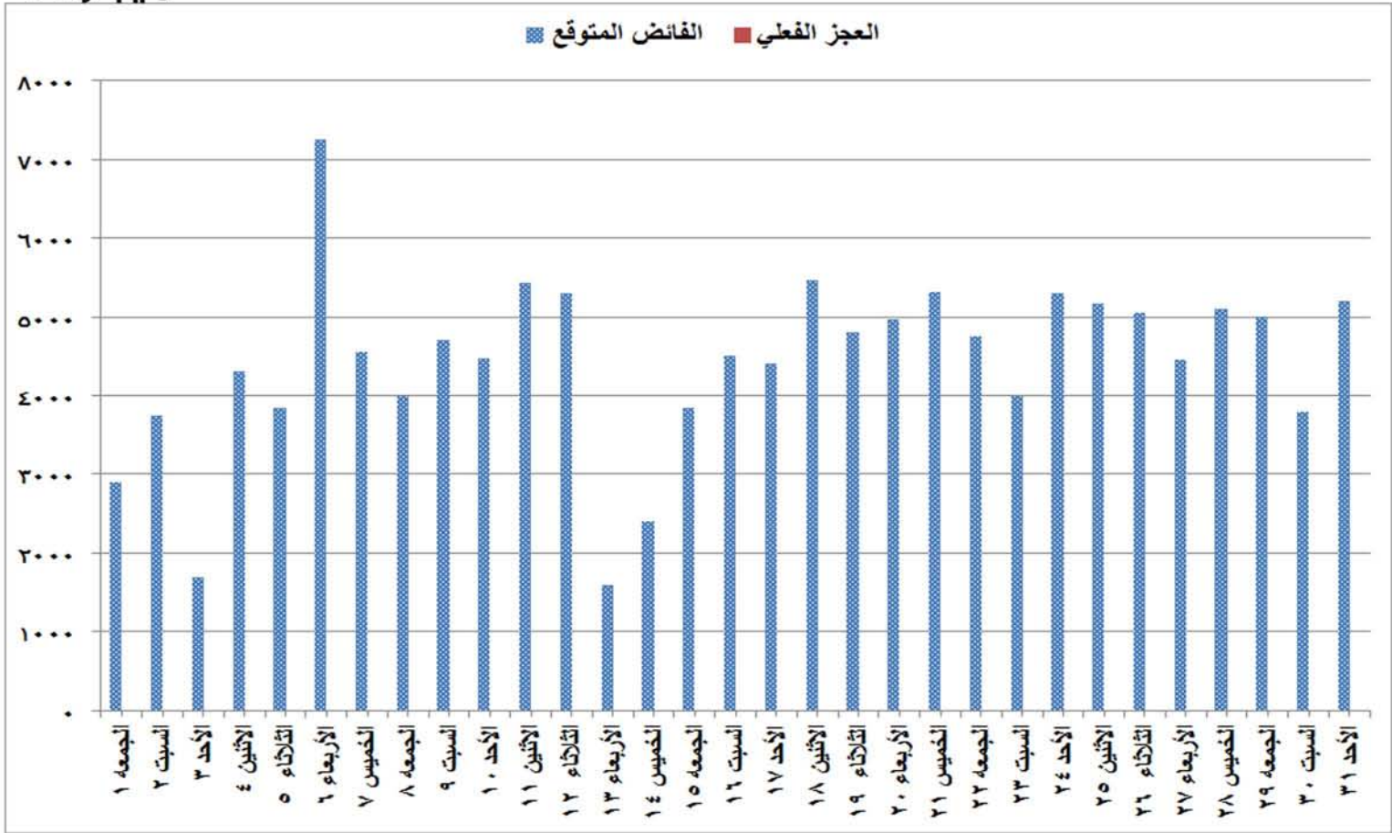
شكل (٧) الفاوض والعجز المتوقع للقدرات خلال شهر يوليو ٢٠١٦
